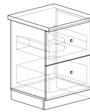
63-60 600x860x600 63-80 800x860x600 63-90 900x860x600 Hettich, орг-я под мойку в комплект не входит
