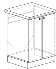
47-60 600x860x600 47-80 800x860x600 47-90 900x860x600 под мойку
